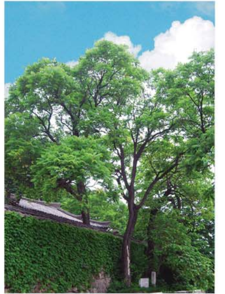
룡악산참중나무
